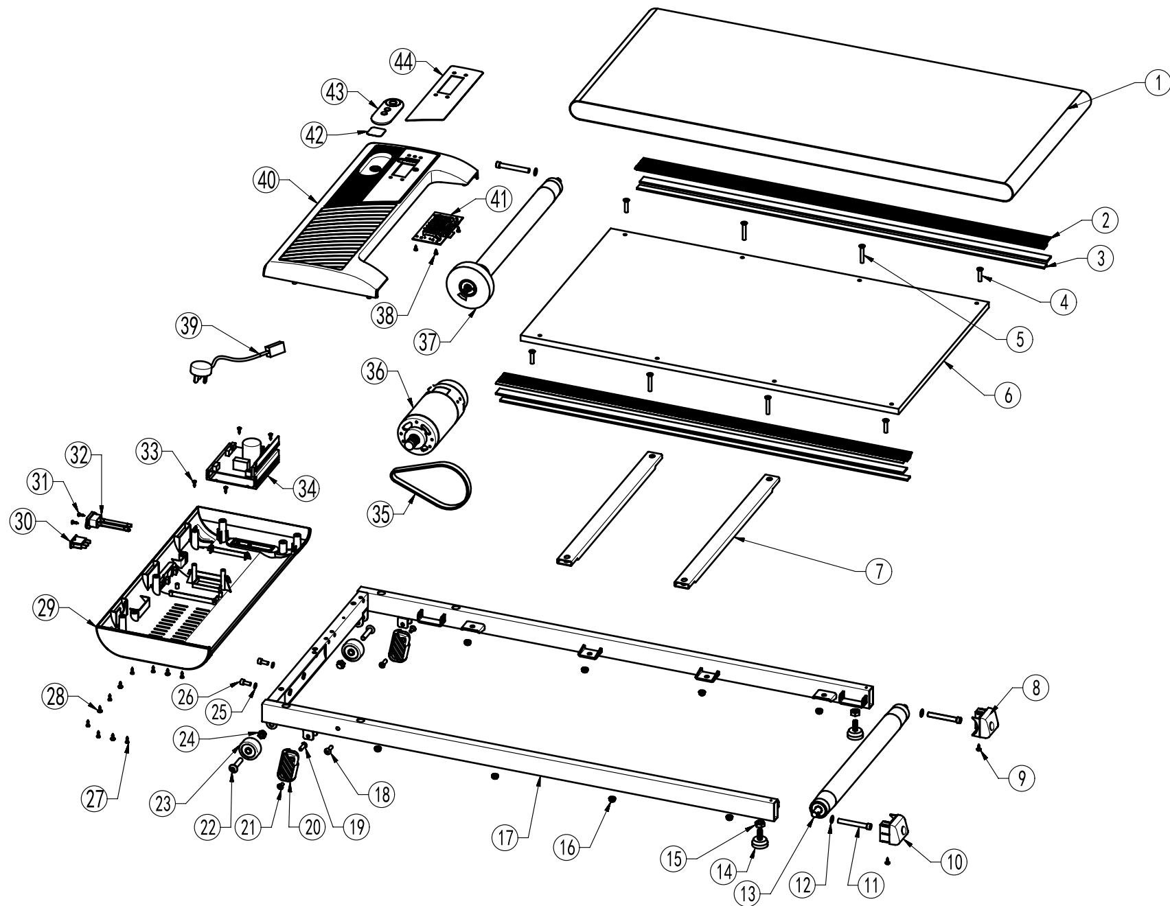
W04G7-爆炸图
