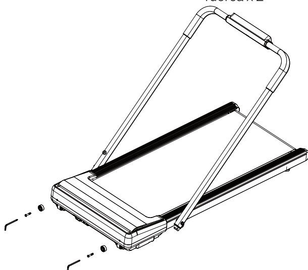
Tuerca de Bloqueo y Tuerca x 2
