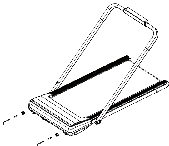
Tapis de pied x 2
